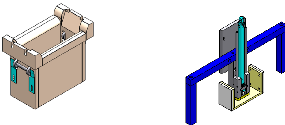
Формоващи части – формоващ джоб и бутало
